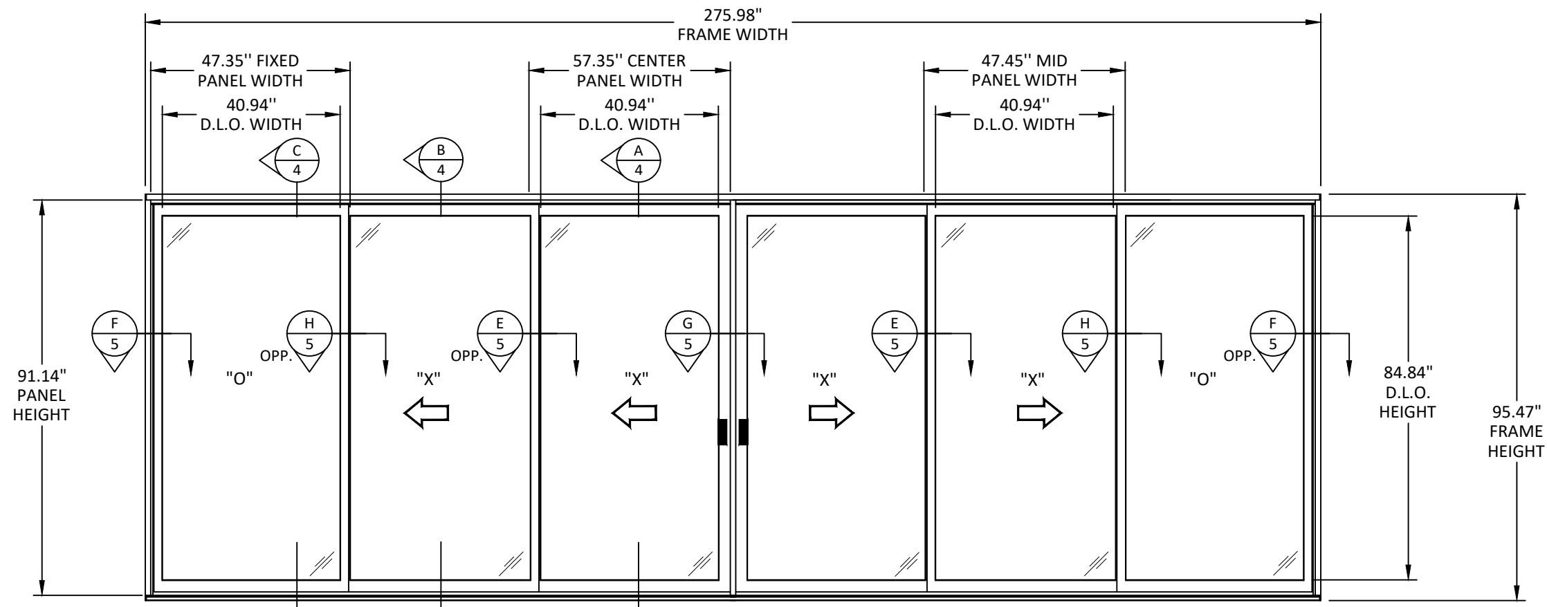
ELEVATION SLIDING DOOR
